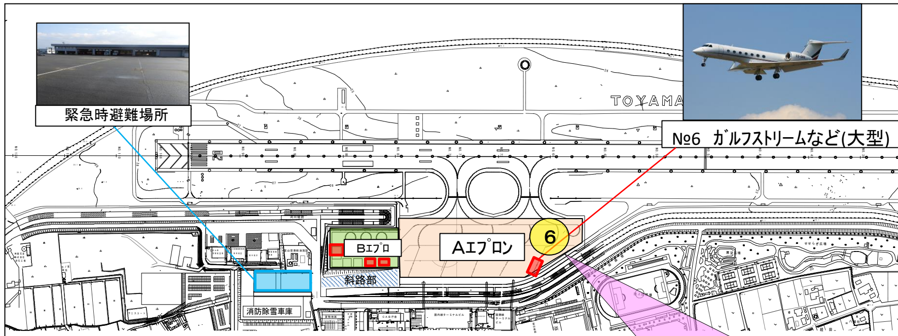
BI7口(拡大図)
